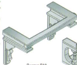
Портал П10 Г - 600 мм В - 700 мм Ш - 1180 мм
