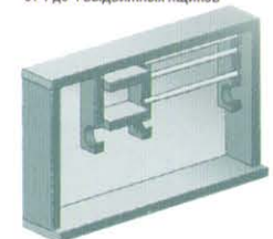
Полка П5-800 Полка П5-600 Г - 250 мм В - 560 мм Ш - 600 (800) мм
